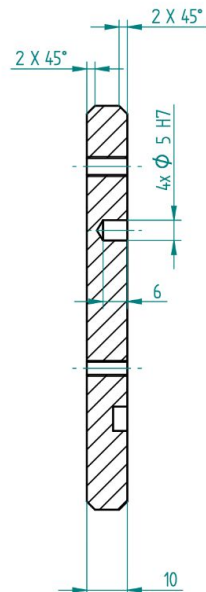
Schnitt A-A
