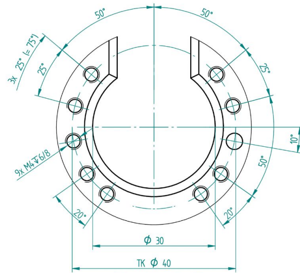
Einzelheit Z 2:1
